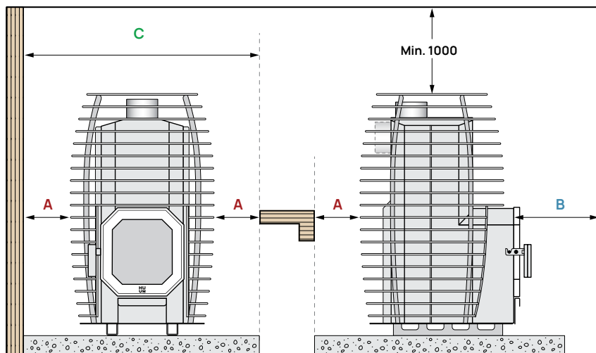
7. attēls. HIVE Flow pirts krāsns drošības attālumi no uzliesmojošiem materiāliem (piemēram, koka sienas, lāvas u. c.).
