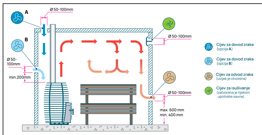
Slika 12. Mehanička ventilacija u sauni u kojoj se koristi peč na drva.
