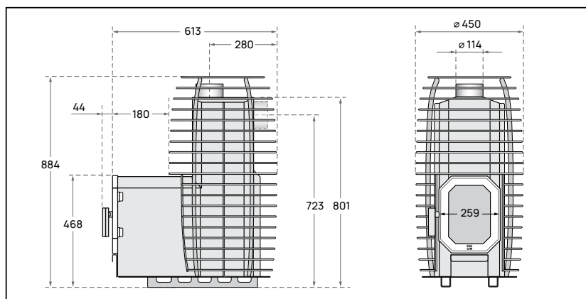
4 pav. Pirties krosnelės HIVE Flow Mini LS matmenys.
