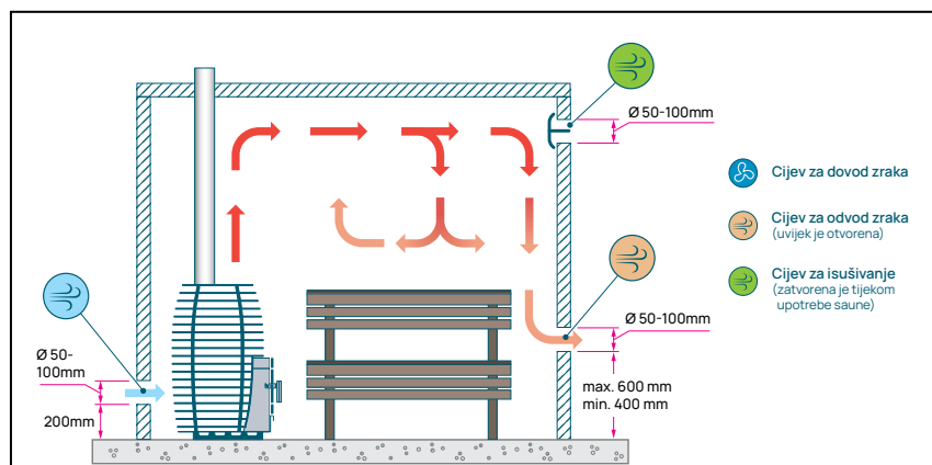
Slika 11. Gravitacijska ventilacija u sauni u kojoj se koristi peč na drva.
