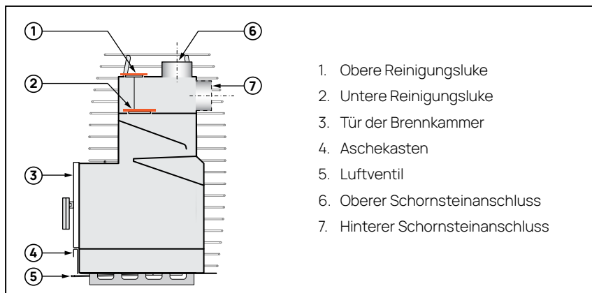
Abbildung 18. Einzelheiten zum HIVE flow Saunaofen
